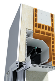
DEMI-LINTEAU OPTIBLOC
