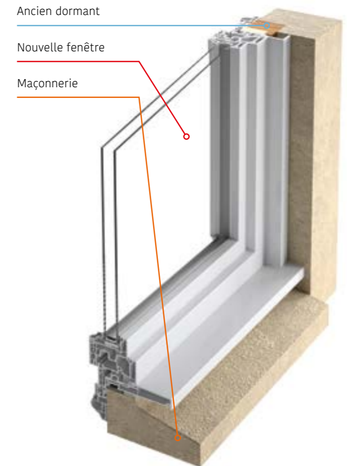
Pose en rénovation avec dépose de l'appui bois
